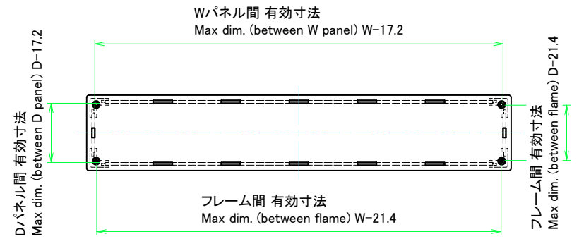
下カバー / Bottom cover
